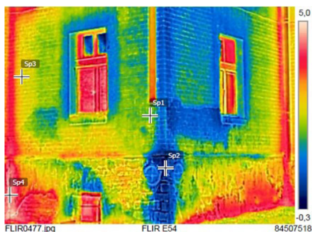
II. 18. Badanie termowizyjne fasad familoków w Bytomiu, Bobrku – narożnik typowego budynku. Lokalne wychłodzenie w miejscu większej ilości elementów metalowych (dobrze przewodzących ciepło), elementy metalowe przyjmują temperaturę otoczenia. Fot. M. Krause-Świerczyńska, 01.2023
