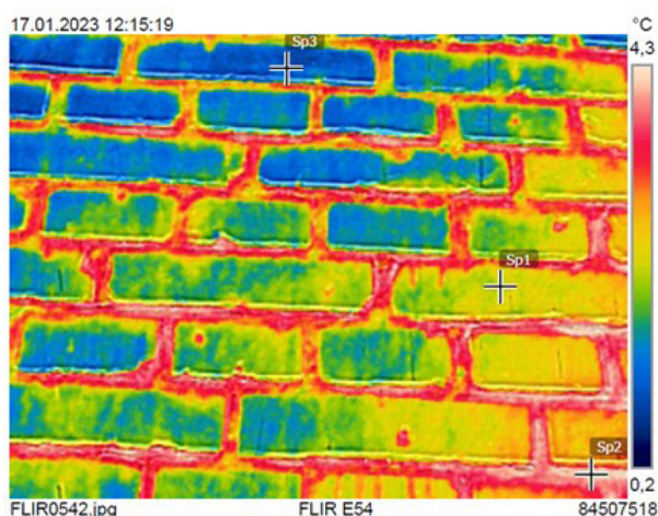
I. II. 17. Badanie termowizyjne fasad familoków w Bytomiu, Bobrku – różnice w izolacyjności cieplnej materiałów przegrody budowlanej, Sp1 = 2,9^{\circ}\text{C} , Sp2 = 4,1^{\circ}\text{C} , Sp3 = 2,5^{\circ}\text{C} . Fot. M. Krause-Świerczyńska, 01.2023
