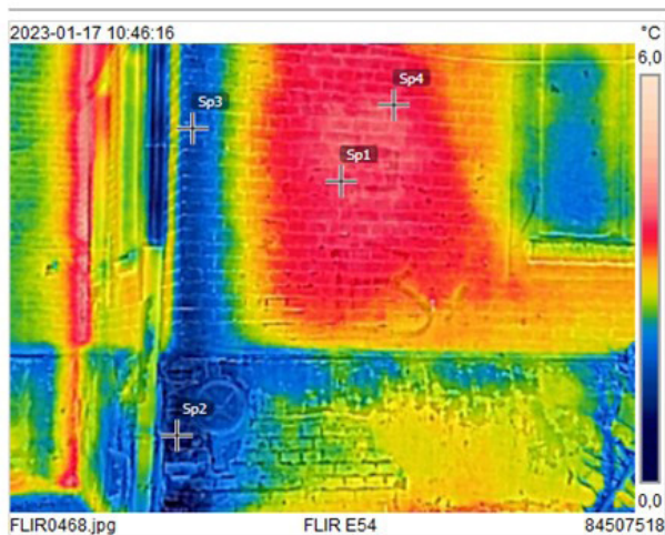
II. 16. Badanie termowizyjne fasad familoków w Bytomiu, Bobrku – widoczny podwójny efekt temperaturowy – silne zawilgocenie i efekt naroża, klatka schodowa nieogrzewwana. Fot. M. Krause-Świerczyńska, 01.2023
