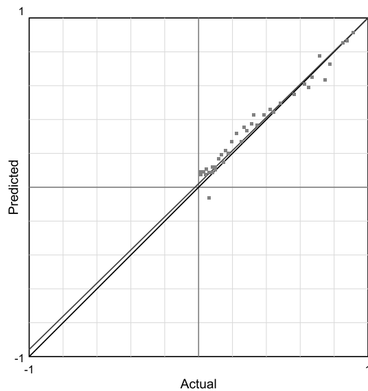
Fig. 15. Regression analysis.
