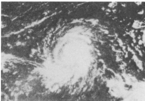
NASA ATS 111 16 AUG 69 1560Z 31B
