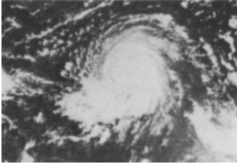
NASA ATS 111 16 AUG 69 1337Z 20B
