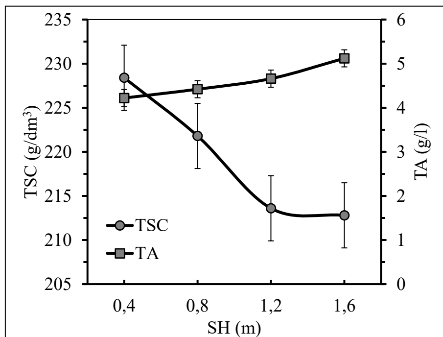
Abbildung 3. Mostgewicht (TSC) und titrierbare Gesamtsäure (TA) im Traubensaft der Rebsorte 'Aromatnyi' ( Vitis vinifera L.) bei verschiedenen SH.
