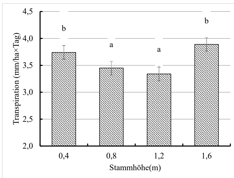
Abbildung 2. Einfluss SH bei der Rebsorte 'Aromatnyi' ( Vitis vinifera L.) auf die Transpirationsrate. Dargestellt sind die Durchschnittswerte für den Zeitraum 2016-2020 \pm SE ( n = 5 ). Laut Duncans Post-hoc-Test ( p \leq 0,05 ) weisen Buchstaben auf signifikante Unterschiede zwischen Varianten hin.
