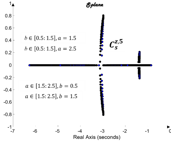
Fig. 12. Root contour k_e = 5
