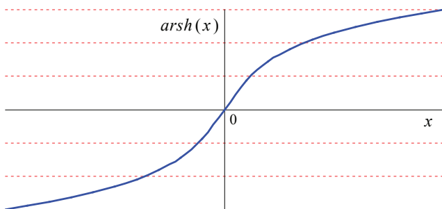
Slika 5: Kriva funkcije \operatorname{arsh}(x)
