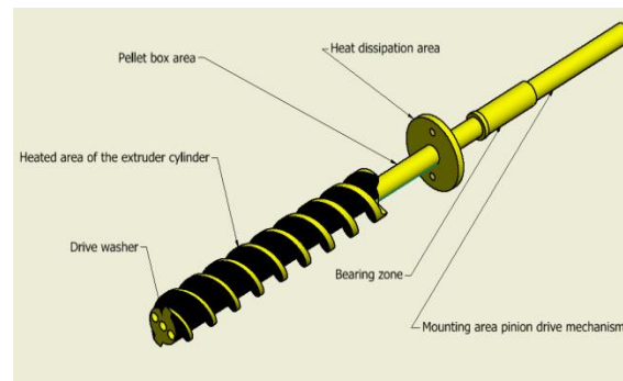
Fig. 4: Conveyor worm[12]
