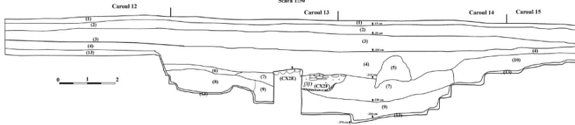
Fig. 7. Profilul de est al carourilor 12 (6x6 m), 13 (6x6 m) și 14 (6x6 m). Scara 1:50. Legenda: (1) vegetal; (2) pământ negru fără materiale arheologice; (3) pământ negru cu materiale arheologice (nivel roman); (4) pământ negru cu pigment galben ce conține materiale arheologice (nivel preistoric) și cu urme de cărbune; (5) groapă: pământ galben cu pigment negru; (6) lentilă de pământ galben; (7) pământ negru afânat cu urme de cărbune și cu oase de animale + materiale arheologice (preistoric); (8) pământ negru amestecat cu galben și cu materiale arheologice (preistoric); (9) pământ galben amestecat cu negru și rar cu materiale arheologice (preistoric); (10) pământ negru afânat cu urme de galben și cu materiale arheologice (preistoric); (11) CX2F: pământ cu cărbune și pigment de lut ars și cu fragmente ceramice (preistoric); (12) CX2E: bucăți de lut ars roșatic cu fragmente ceramice (preistoric); (13) steril arheologic: argilă galbenă nisipoasă.
