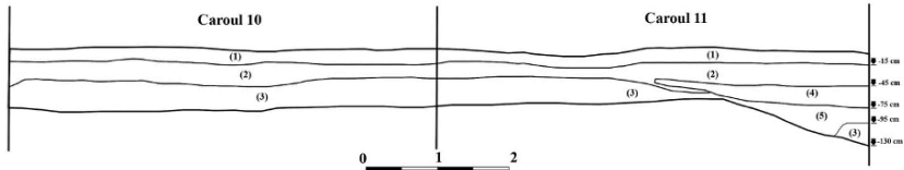
Fig. 6. Profilul de est al carourilor 10 (6x6 m) și 11 (6x6 m). Scara 1:50. Legenda: (1) vegetal; (2) pământ negru fără materiale arheologice; (3) steril arheologic: argilă galbenă nisipoasă; (4) strat de cultură: pământ negru cu materiale arheologice (nivel preistoric); (5) pământ maroniu fără materiale arheologice.
