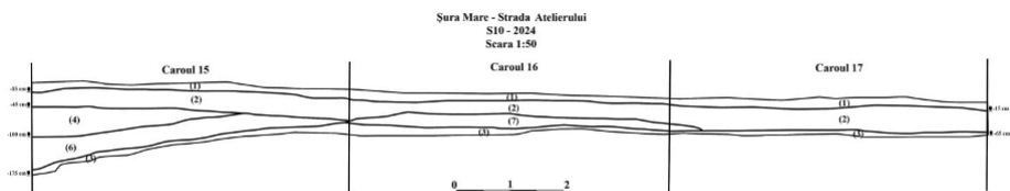
Fig. 8. Profilul de est al carourilor 15 (6x6 m), 16 (6x6 m) și 17 (6x6 m). Scara 1:50.
