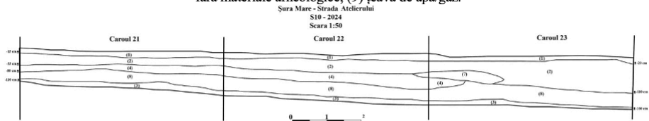
Fig. 10. Profilul de est al carourilor 21 (6x6 m), 22 (6x6 m) și 23 (6x6 m). Scara 1:50.
