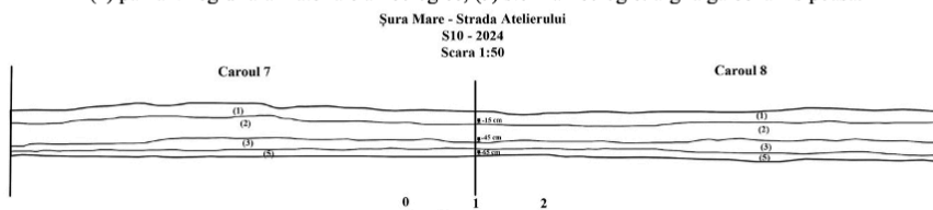
Fig. 4. Profilul de est al carourilor 7 (7x7 m) și 8 (7x7 m). Scara 1:50. Legendă: (1) vegetal; (2) pământ negru cu rar materiale arheologice; (3) pământ maroniu fără materiale arheologice; (5) steril arheologic: argilă galbenă nisipoasă.
