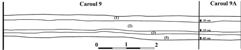
Fig. 5. Profilul de est al carourilor 9 (7x7 m) și 9A (1.5x6 m). Scara 1:50. Legendă: (1) vegetal; (2) pământ negru cu rar materiale arheologice; (3) pământ maroniu fără materiale arheologice; (5) steril arheologic: argilă galbenă nisipoasă.
