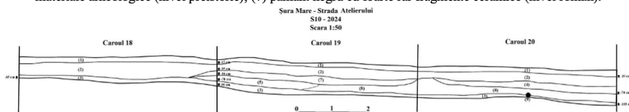
Fig. 9. Profilul de est al carourilor 18 (6x6 m), 19 (6x6 m) și 20 (6x6 m). Scara 1:50.
