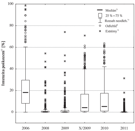
Obr. 3. Intenzita poškození smrkových porostů sněhem v letech 2006–2011 (X/2009 = sněhový polom z října 2009; v roce 2007 byly škody zanedbatelné a intenzita nebyla vyhodnocena) Fig. 3. Intensity of snow damage to Norway spruce stands during 2006–2011 (X/2009 = snow damage in October 2009; damage was negligible in 2007 and intensity was not evaluated).
