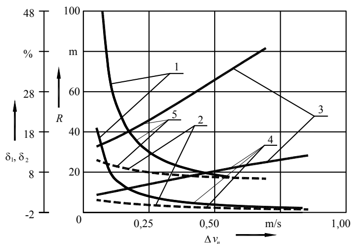
Рисунок 1. Зависимость радиуса поворота (кривые 1) и буксования отстающей (кривые 2) и забегающей (кривые 3) гусениц от \Delta v_n при движении со скоростью 7 км·ч -1 без крюковой нагрузки (кривые 4) и с нагрузкой 40 кН (кривые 5)
