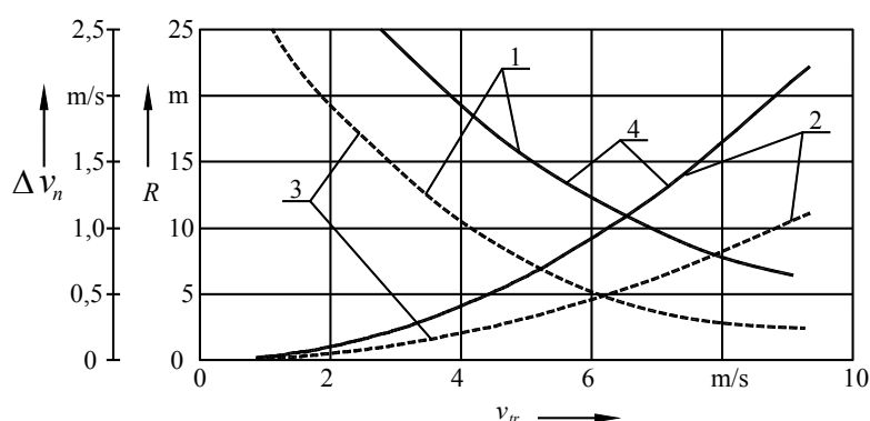
Рисунок 2. Зависимости предельного значения по заносу \Delta v_n (кривые 1) и радиуса поворота (кривые 2) от скорости движения на влажной почве при \mu=0,4 (кривые 3) и на сухой почве \mu=0,8 (кривые 4)
