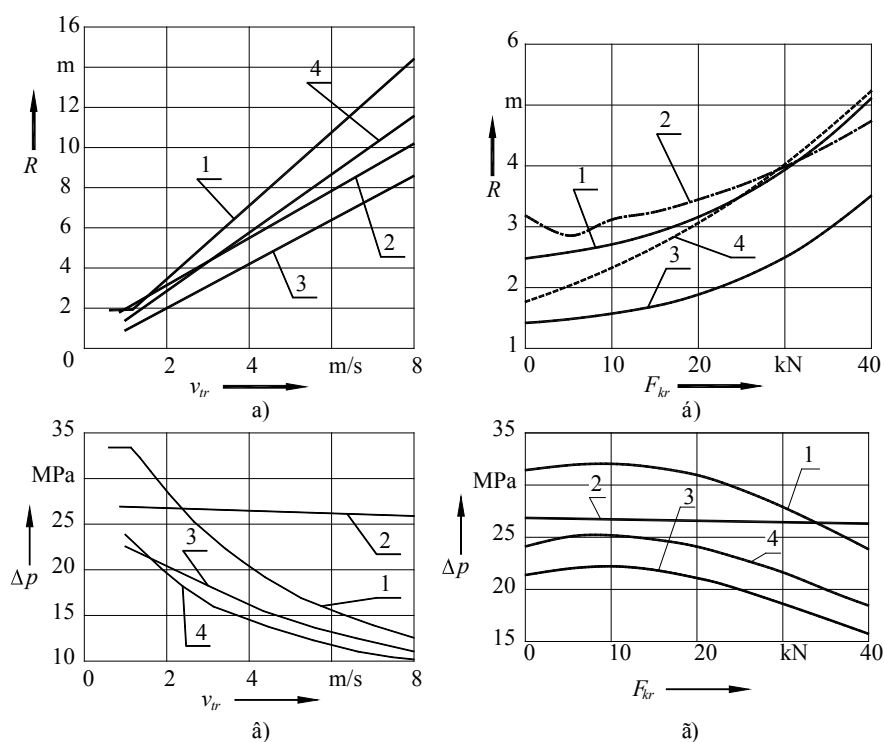
Рисунок 3. Зависимость радиуса поворота R и давления рабочей жидкости в ОГП \Delta p от скорости движения v_{tr} и крюковой нагрузки F_{kr} : цифрами обозначены номера схем в соответствии таблицей 2
