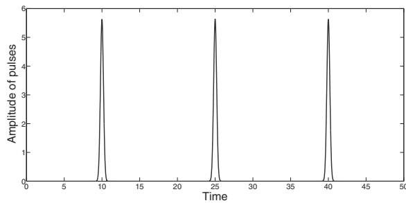
Fig. 2. Gaussian pulses (4) for parameter setting (P1).
