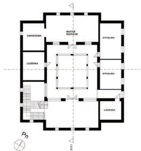
Rzut I piętra skala 1:200
