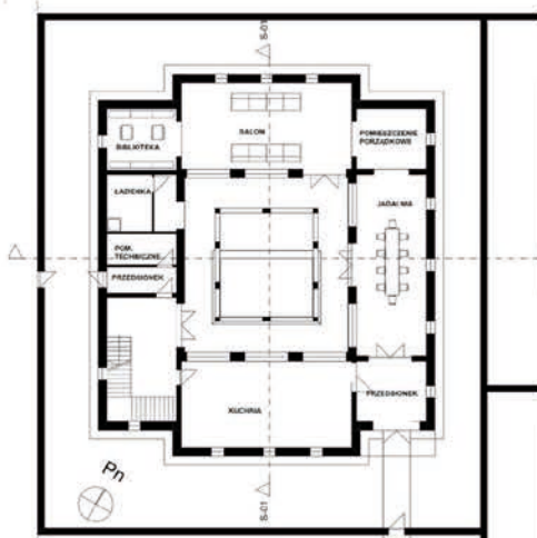
Rzut parteru skala 1:200
