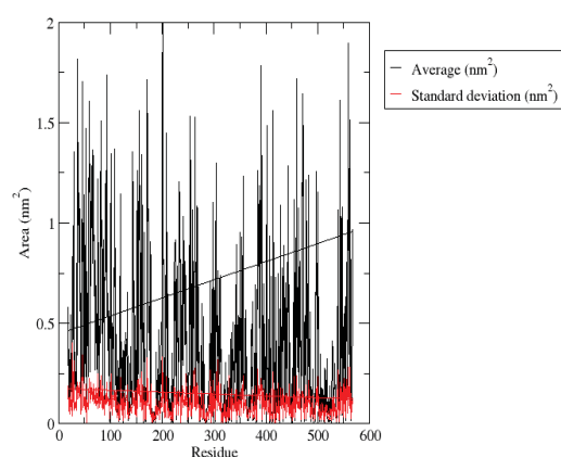
Area per residue over the trajectory
