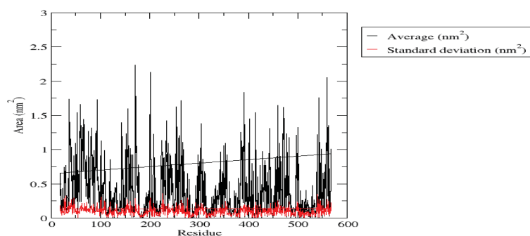
Area per residue over the trajectory
